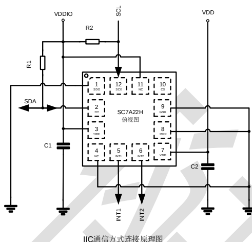
IIC通信方式连接原理图
