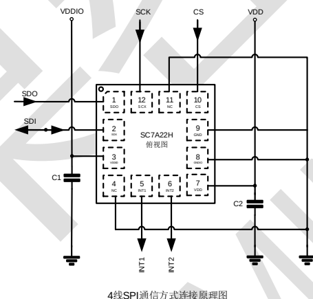
4线SPI通信方式连接原理图
