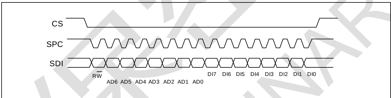
SPI写协议
