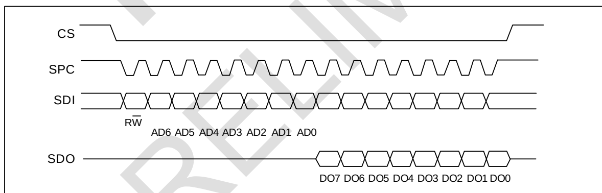
SPI读协议
