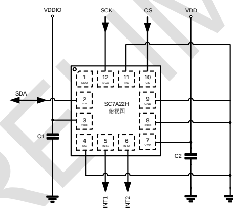
3线SPI通信方式连接原理图
